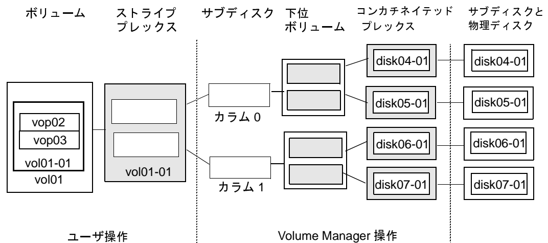
図 21. ストライピングおよびミラーリングした階層化ボリュームの例
