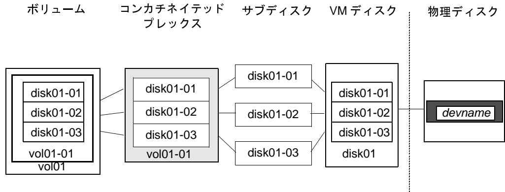
図 11. コンカチネーション構成内のボリュームの例
