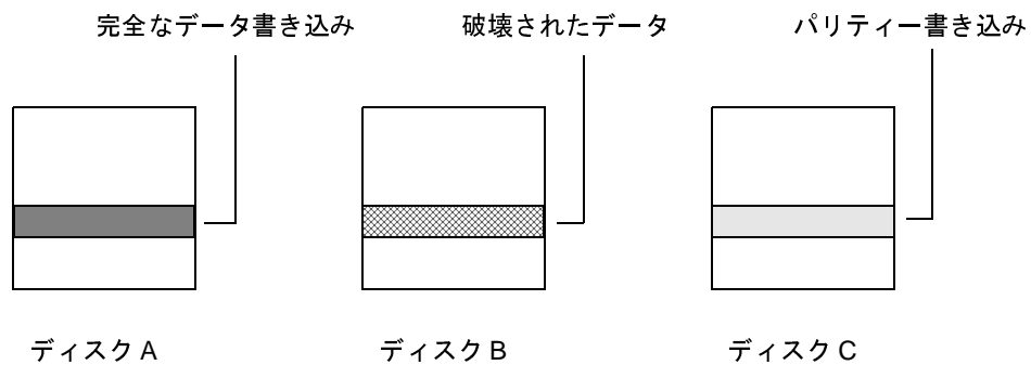
図 20. 不完全な書き込み
