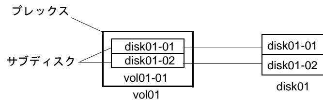
図 6. 2 つのサブディスクから成るプレックスの例
