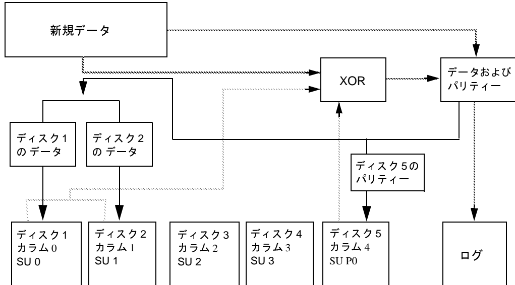
図 27. 読み取り - 変更 - 書き込み
