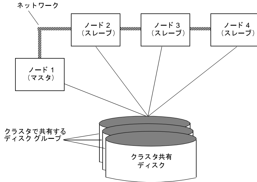
図 24. 4つのノードで構成されるクラスタの例
