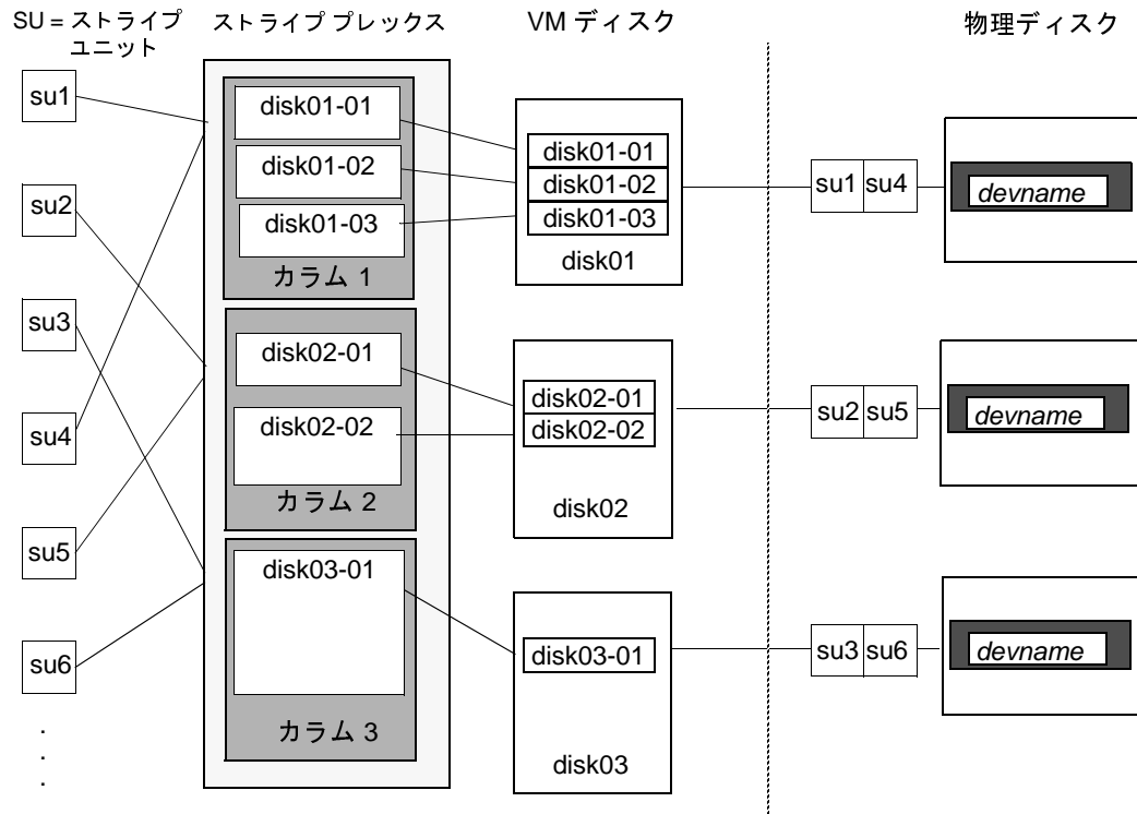
図 15. カラムごとにコンカチネイテッド サブディスクを含むストライプ ブレックスの例
