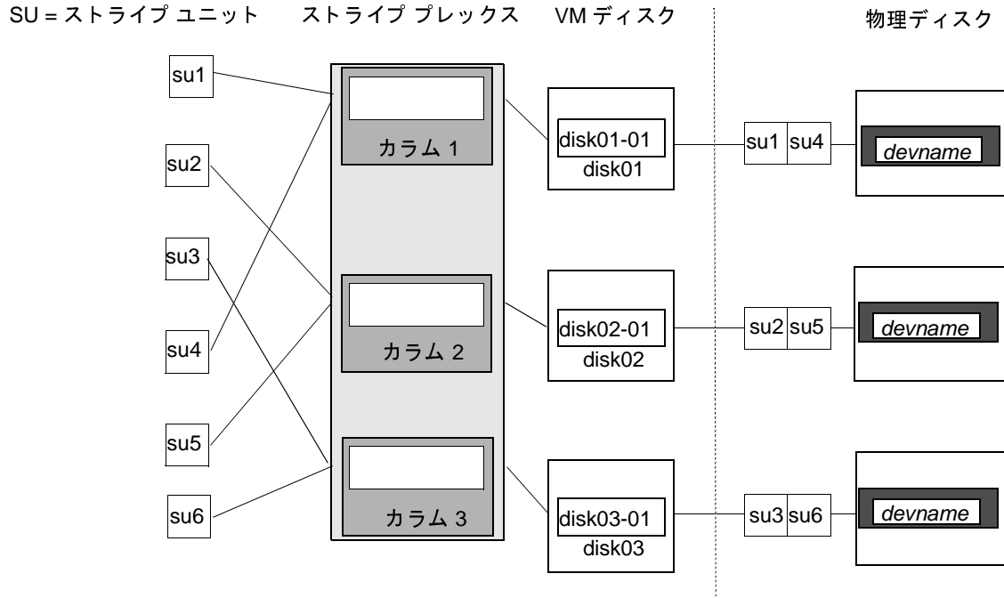
図 14. カラムごとに1つのサブディスクを含むストライププレックスの例
