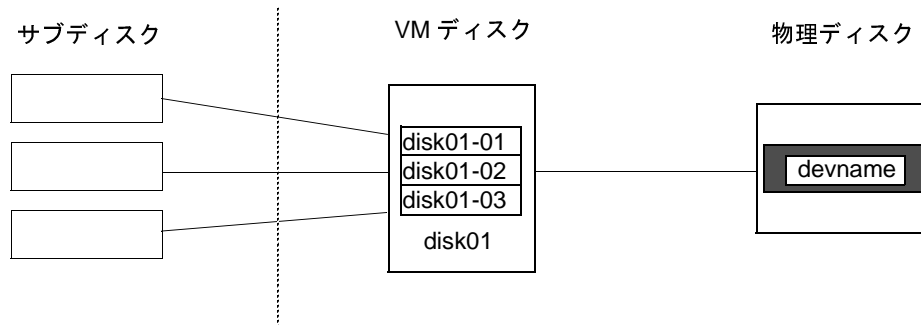
図 5. 1つのVM ディスクに割り当てられた3つのサブディスクの例
