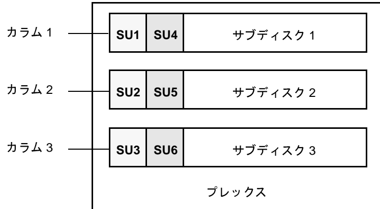
図 13. 3つのディスク（カラム）にわたるストライピング
