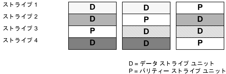
図 16. RAID-5 モデルでのパリティの配置
