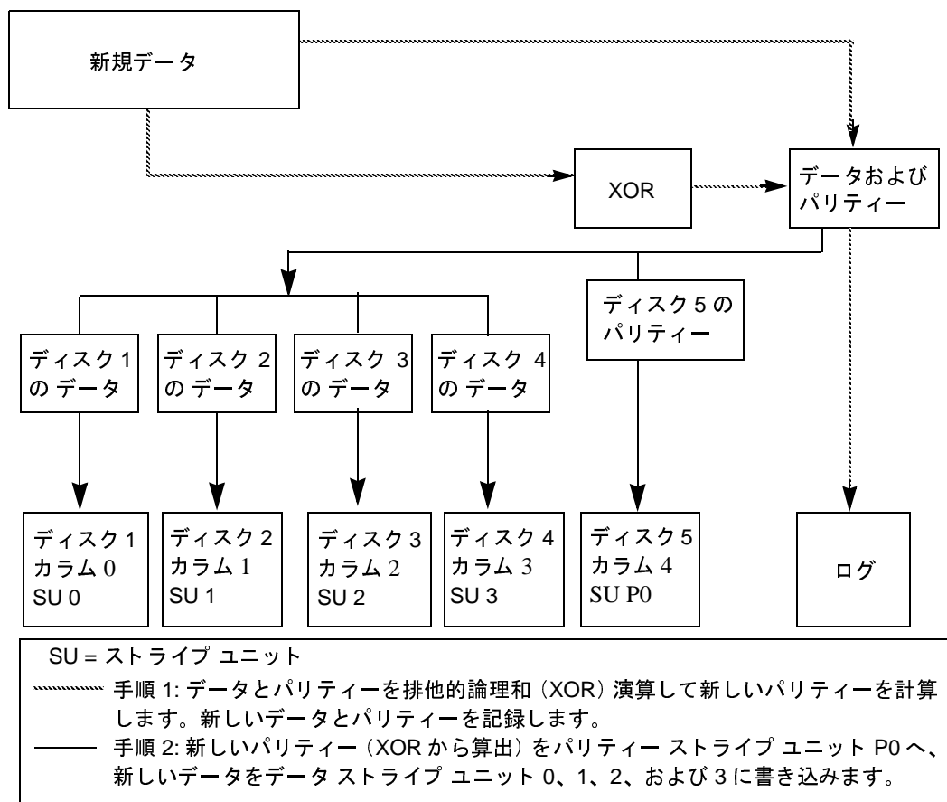
図 28. 全ストライプ書き込み
