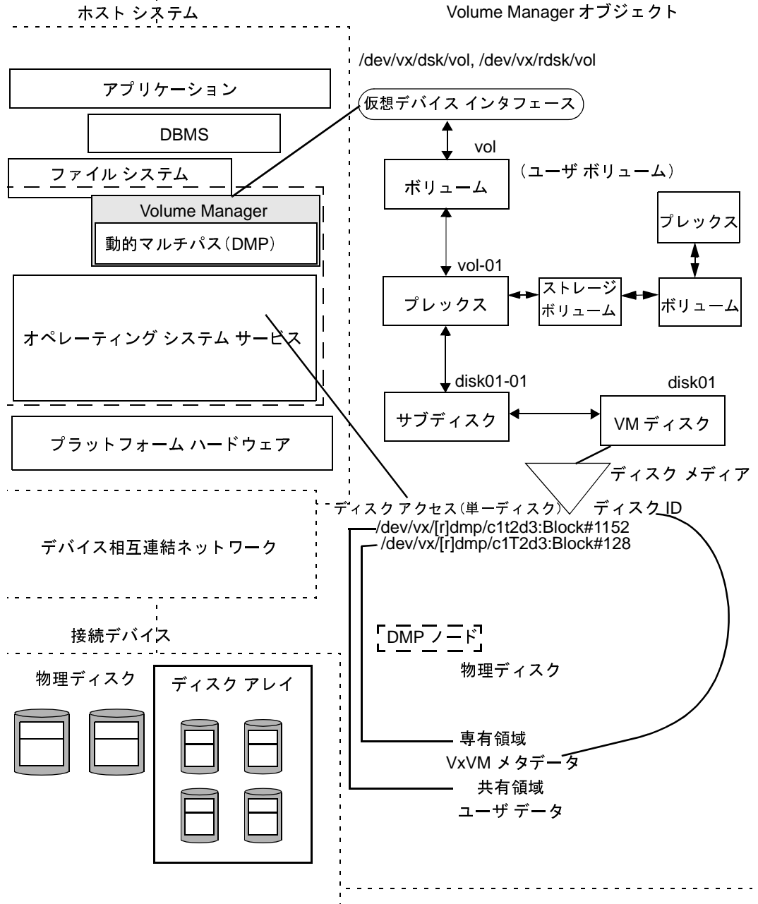
図 22. Volume Manager システムの概念
