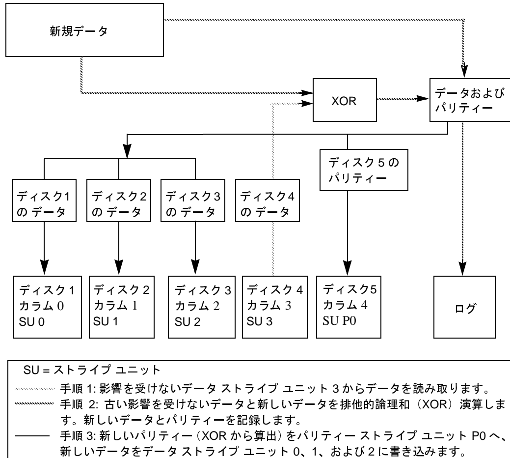
図 29. 復元書き込み
