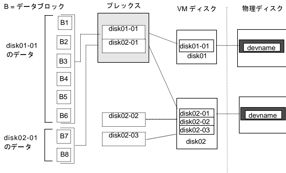
図 12. スパンニングの例
