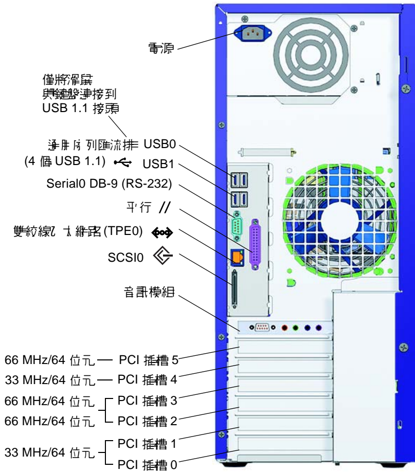
圖 1-4 後面板概觀
