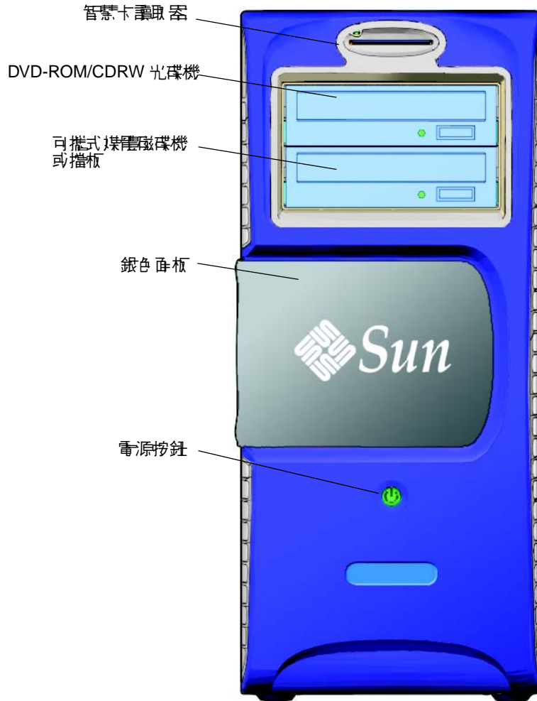
圖 1-3 前面板概觀
