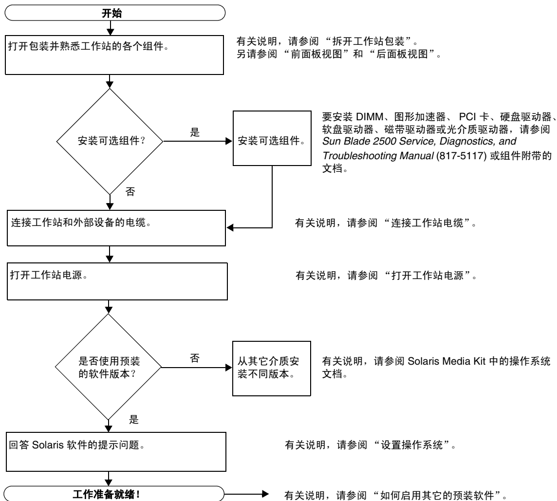
图 1-1 安装下列工作站的过程：Sun Blade 2500 Workstation
