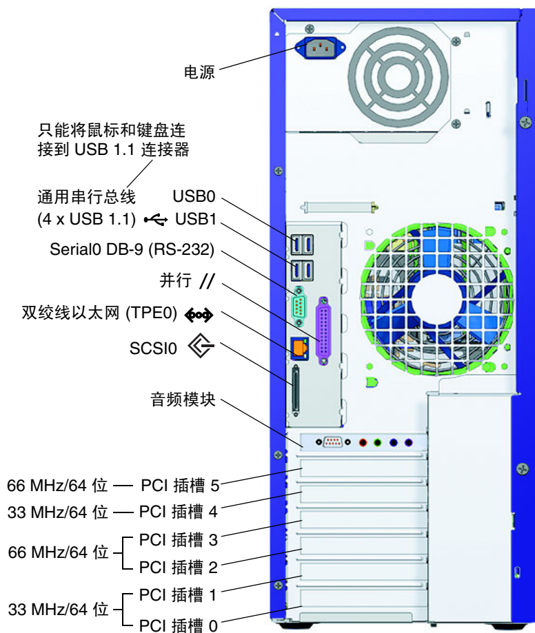
图 1-4 后面板视图
