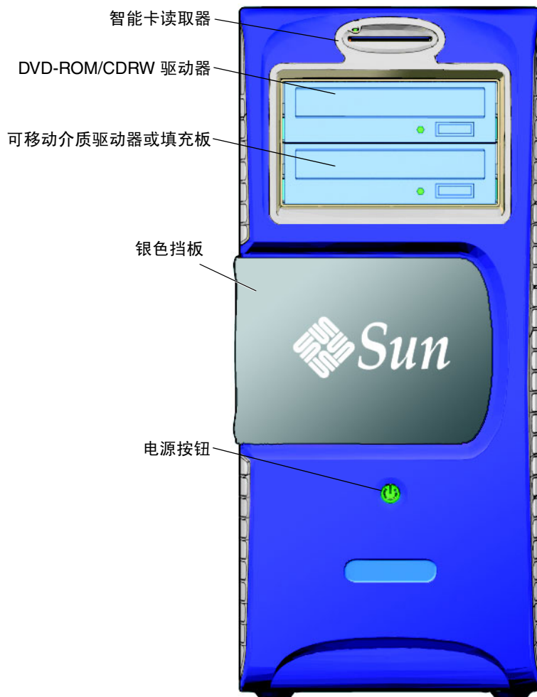
图 1-3 前面板视图
