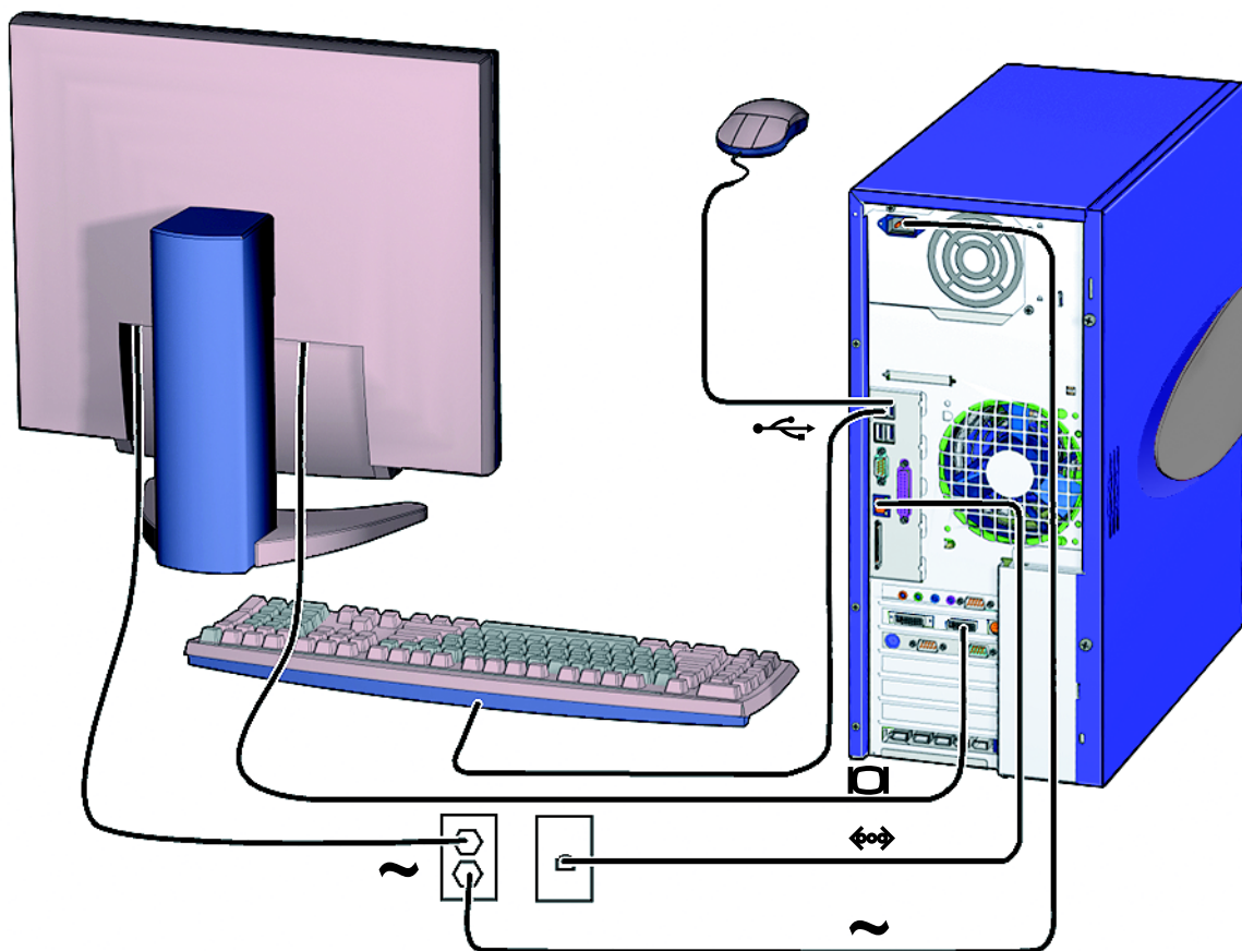
图 1-6 连接下列工作站电缆：Sun Blade 2500 Workstation
