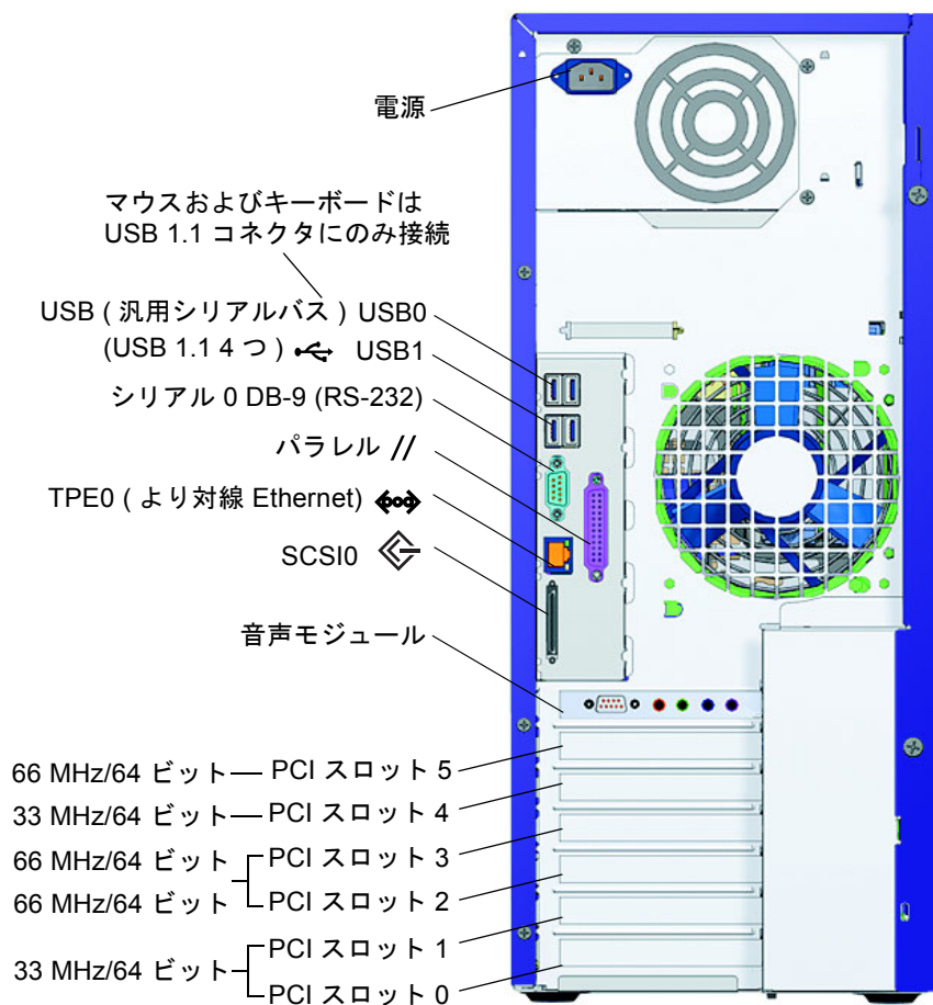
図 1-4 背面パネルの概要
