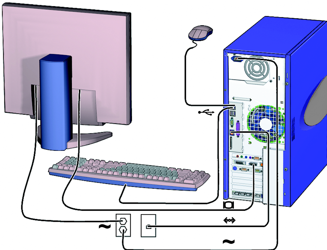
図 1-6 Sun Blade 2500 ワークステーションのケーブル接続
