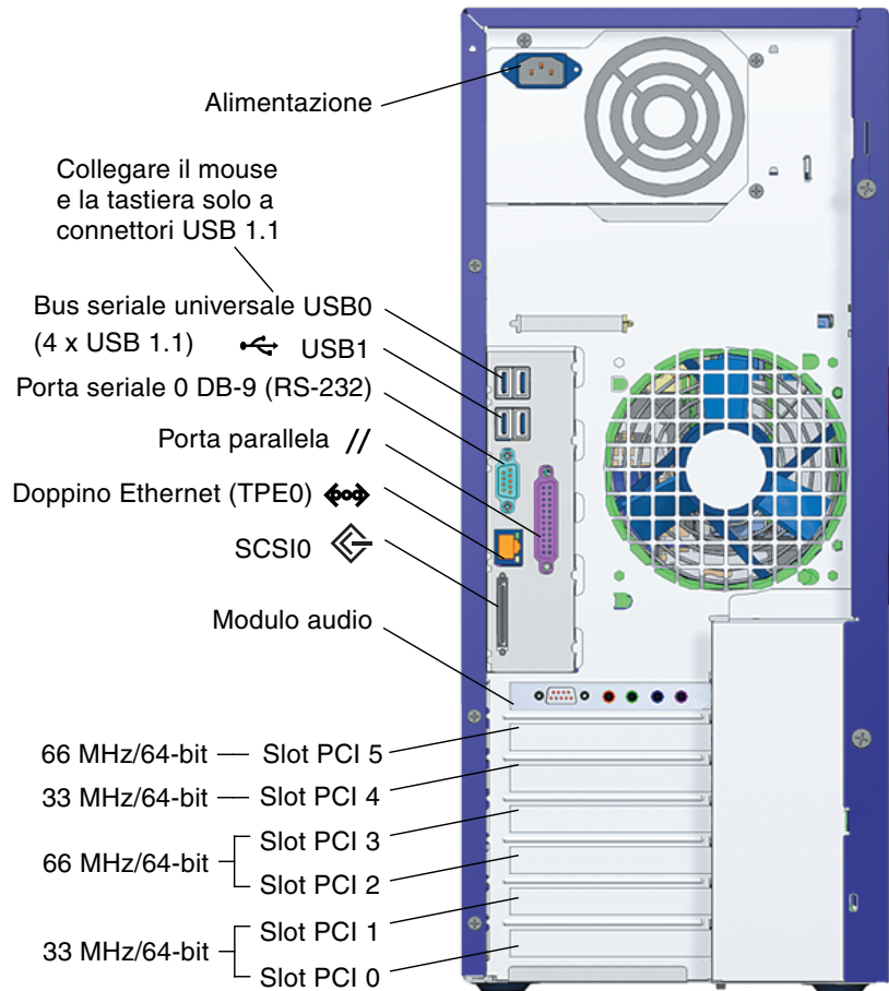
FIGURA 1-4 Pannello posteriore
