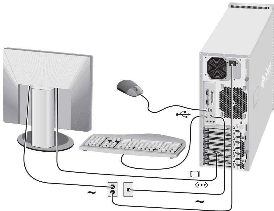
图 1-4 电缆布线
