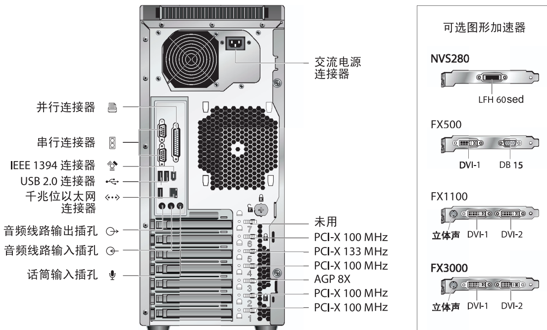
图 1-3 背面板
