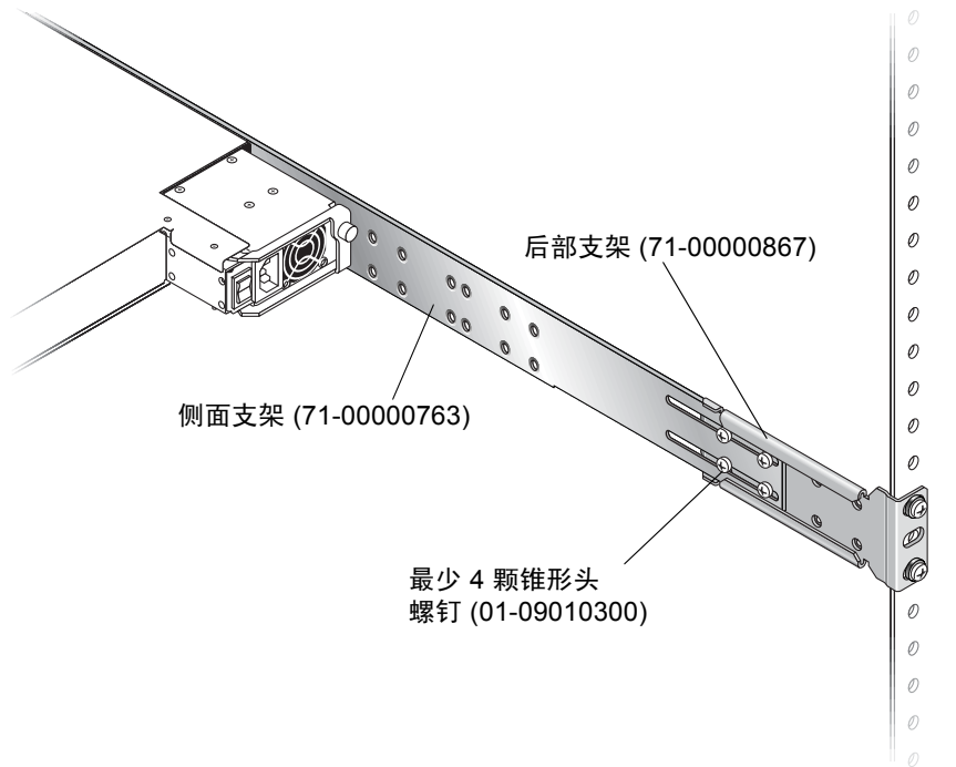
图 2-7 已组装好的后部和侧面支架示例
