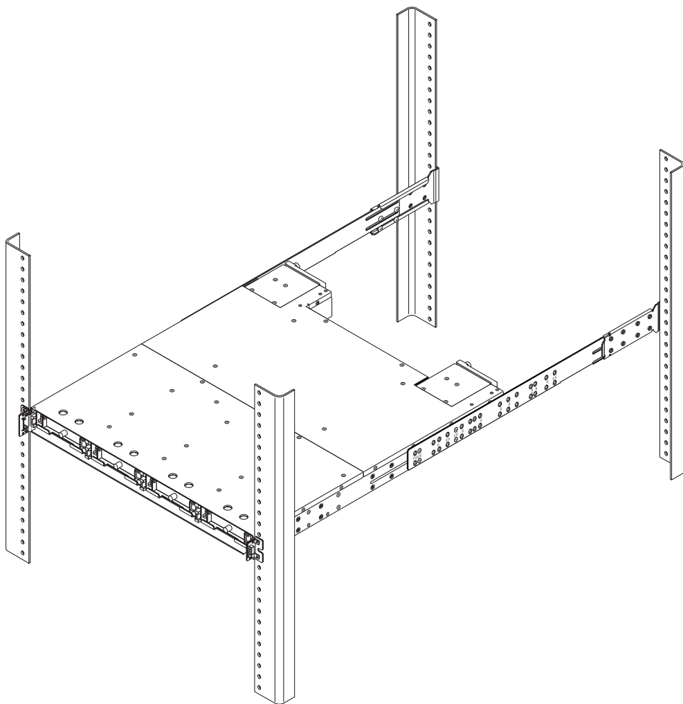
图 2-1 用后支架安装完成之后，不带机箱帽和前盖、通过机架安装的机柜阵列
