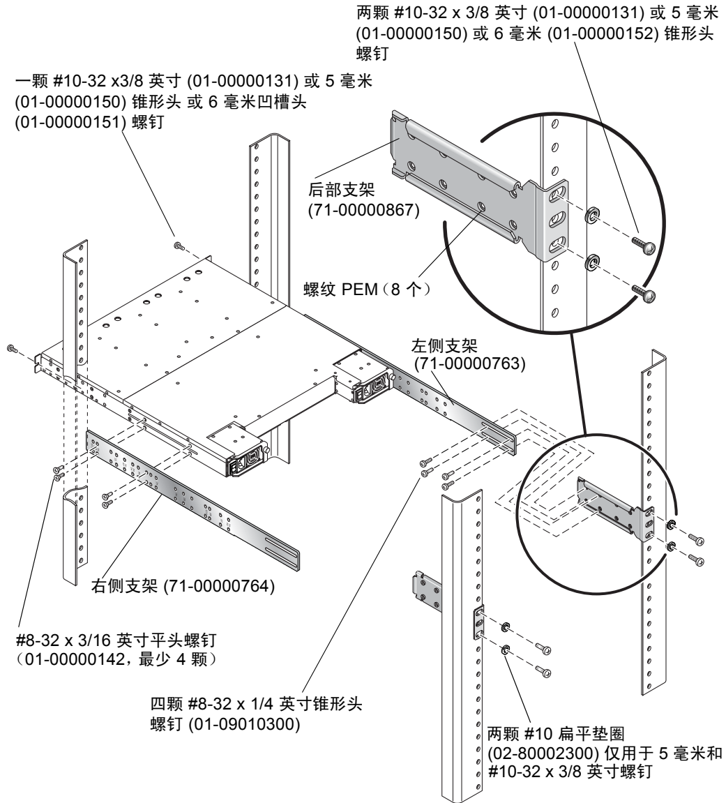
图 2-4 使用后支架的机柜机架安装
