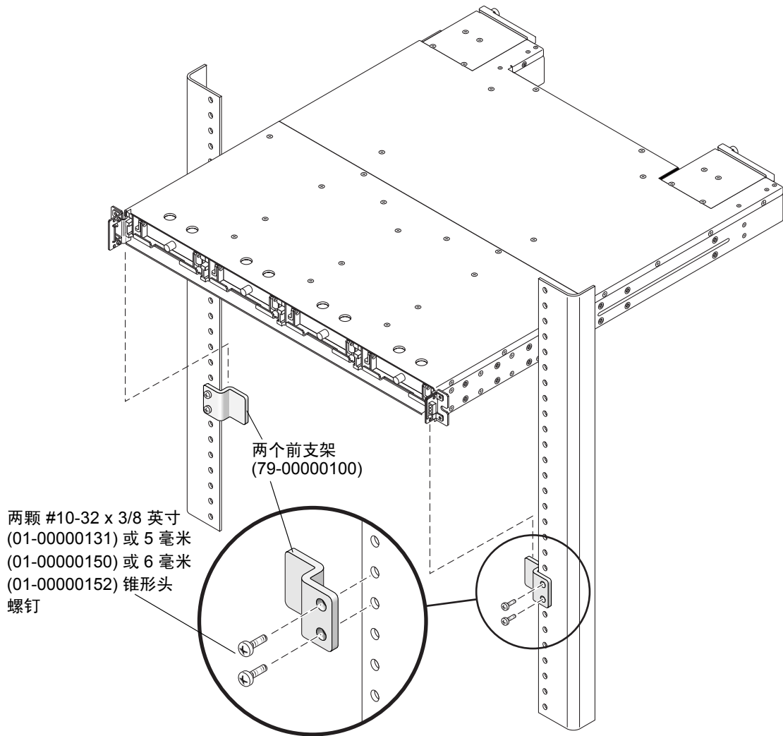
图 2-8 机架前面板上的前支架位置
