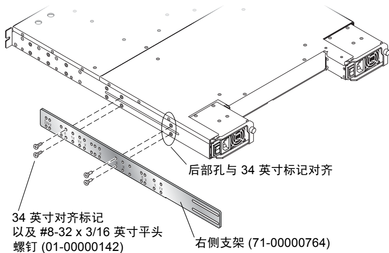
图 2-6 将侧面支架与阵列侧面上的后部螺纹孔对齐
