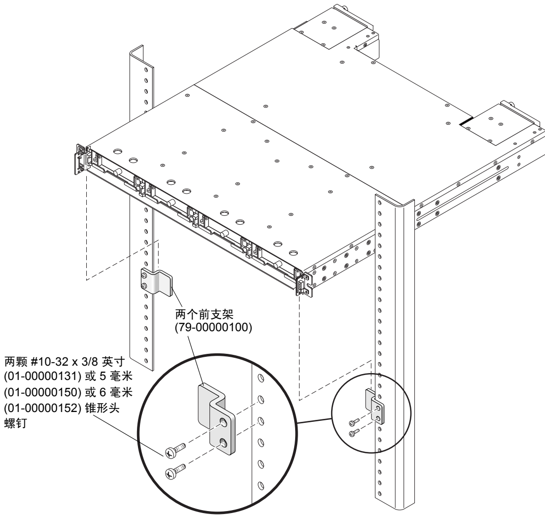
图 2-3 机架前面板上的前支架位置
