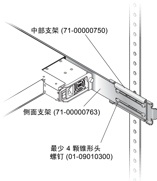
图 2-12 已组装好的中部和侧面支架
