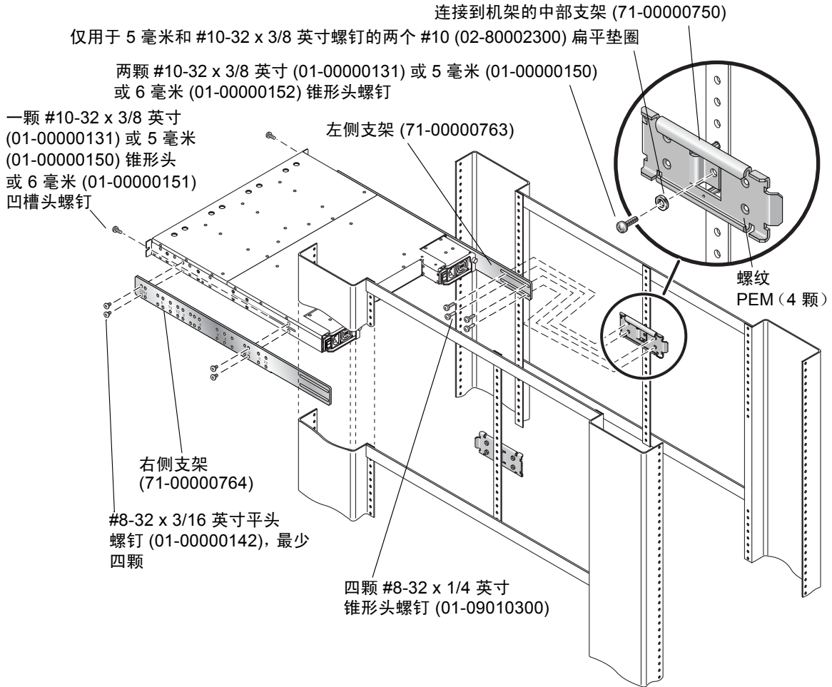
图 2-9 机柜中部支架的机架安装
