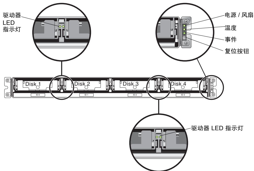
图 4-1 LED 指示灯所在的前面板
