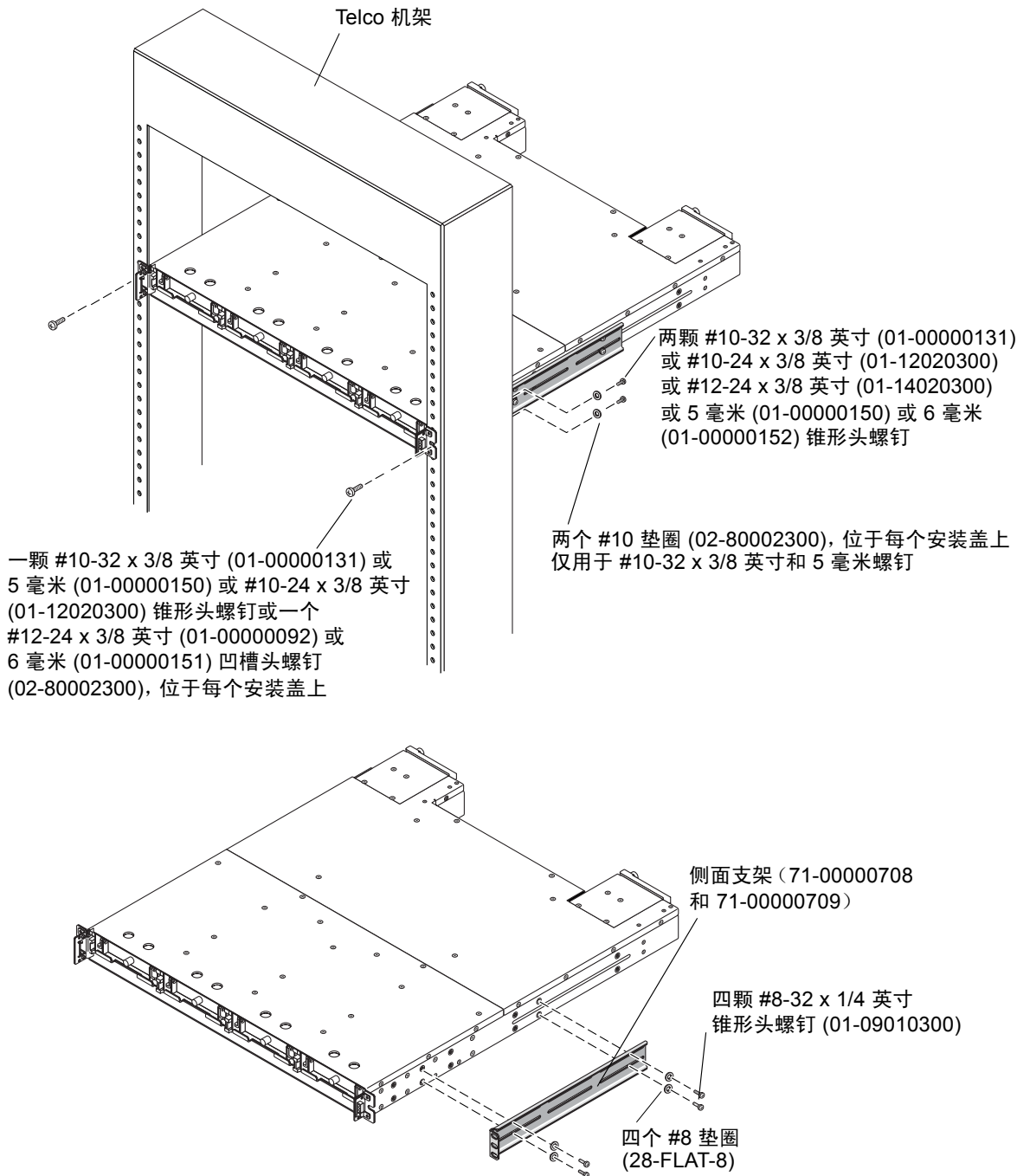
图 3-1 平镶安装装配示例
