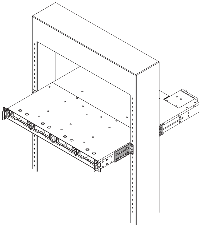
图 3-2 在机架上安装好的 Telco 阵列，未装机箱安装盖和挡板
