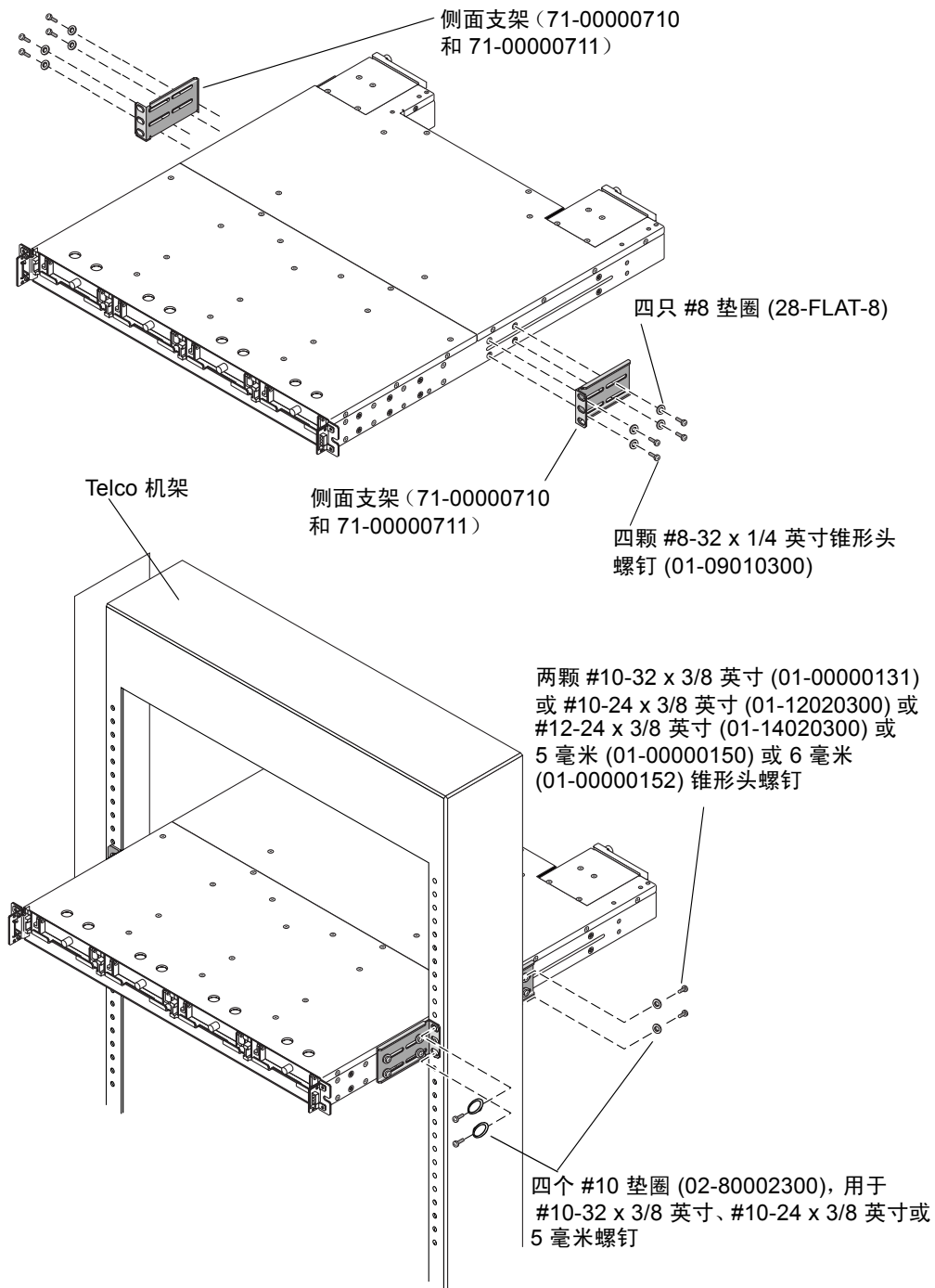
图 3-3 重心安装
