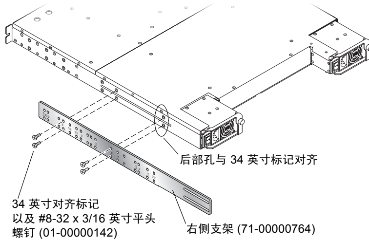
图 2-11 将侧面支架与阵列侧面上的后部螺纹孔对齐
