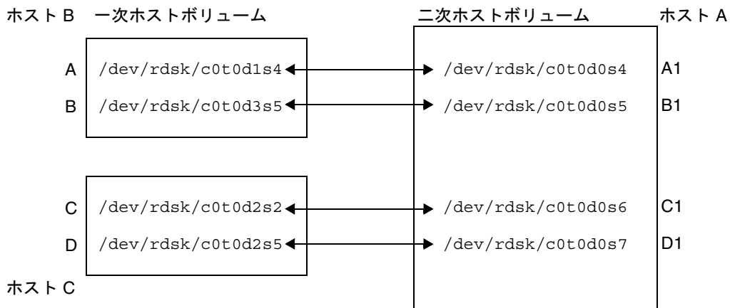
図 2-6 多対 1 のボリュームセットの複製
