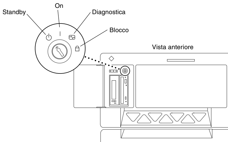
FIGURA 5-1 Posizione degli interruttori a chiave sui sistemi Sun Enterprise 6x00, 5x00, 4x00, 3x00
