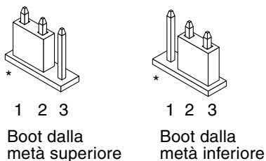
FIGURA 4-6 Impostazione del jumper di controllo del boot per l'esecuzione del boot dalla metà inferiore o dalla metà superiore
