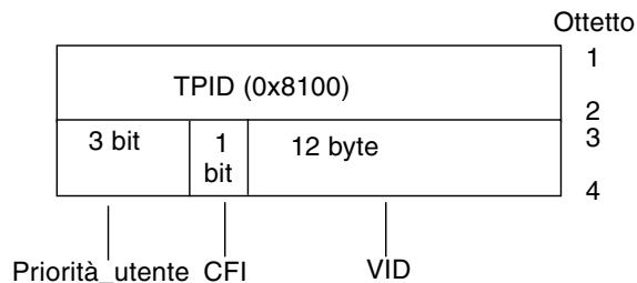
FIGURA 2-1 Formato Ethernet Tag Header
