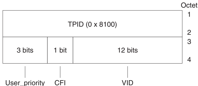
FIGUR 3-1 Ethernet-huvudmärkesformat
