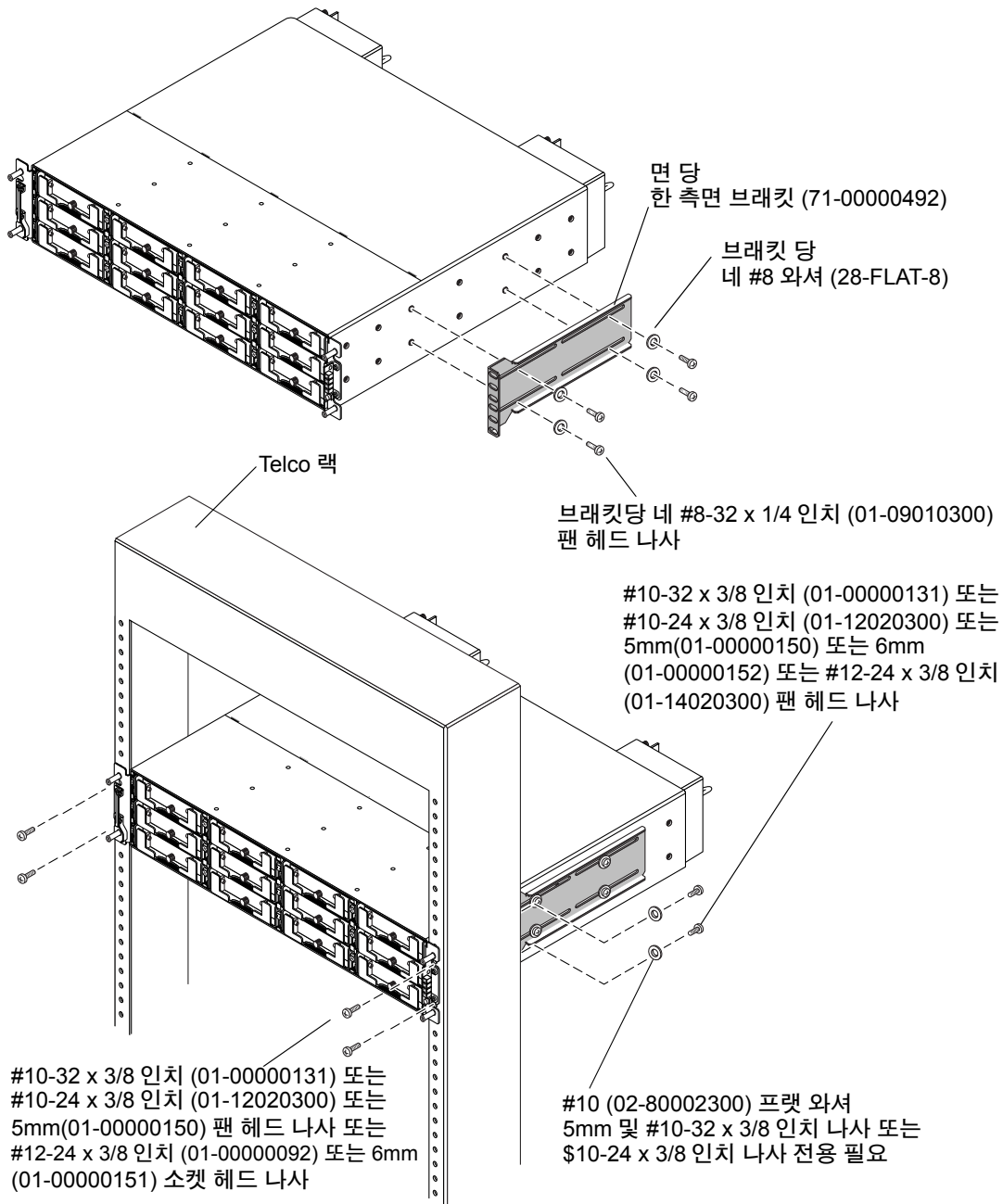
그림 3-1 플러시마운트 조립
