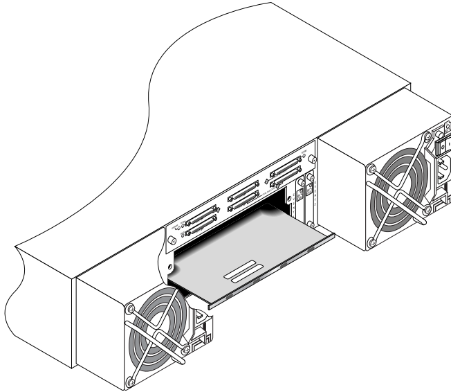
FIGURE 6-1 Module de terminaison partiellement désengagé du châssis
