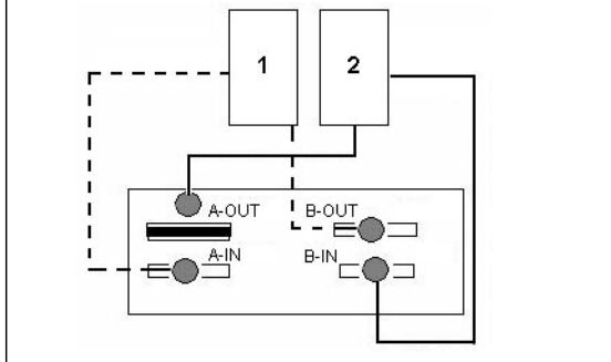
FIGURE 6-6 Suppression d'un seul câble d'un port OUT dans une configuration à deux hôtes
