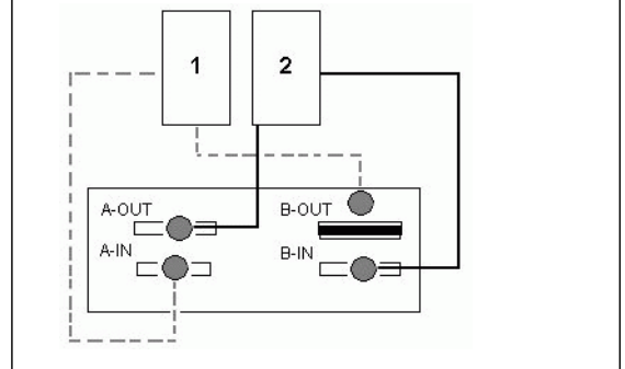
FIGURE 6-6 Suppression d'un seul câble d'un port OUT dans une configuration à deux hôtes
