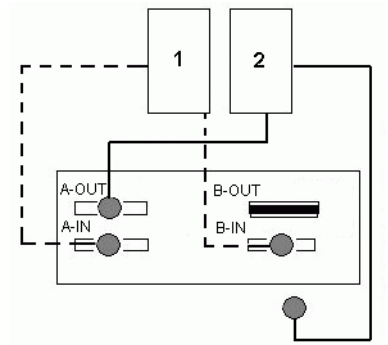
FIGURE 6-5 Débranchement d'un câble simple d'un port IN dans une configuration à deux hôtes
