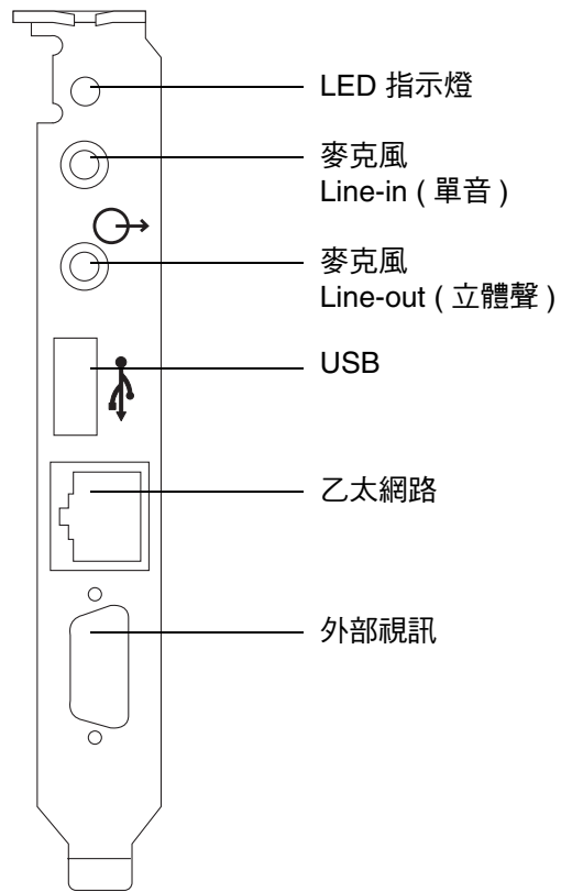
■ 10-1 SunPCi III 主卡的背板接頭
