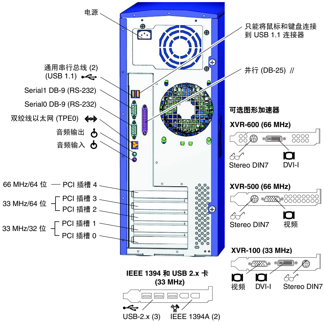
图 1-4 后面板视图
