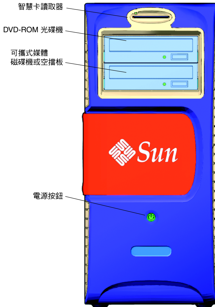
圖 1-3 前面板概觀
