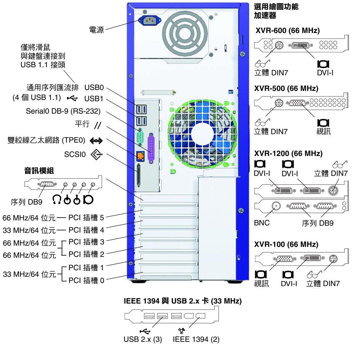
圖 1-4 後面板概觀
