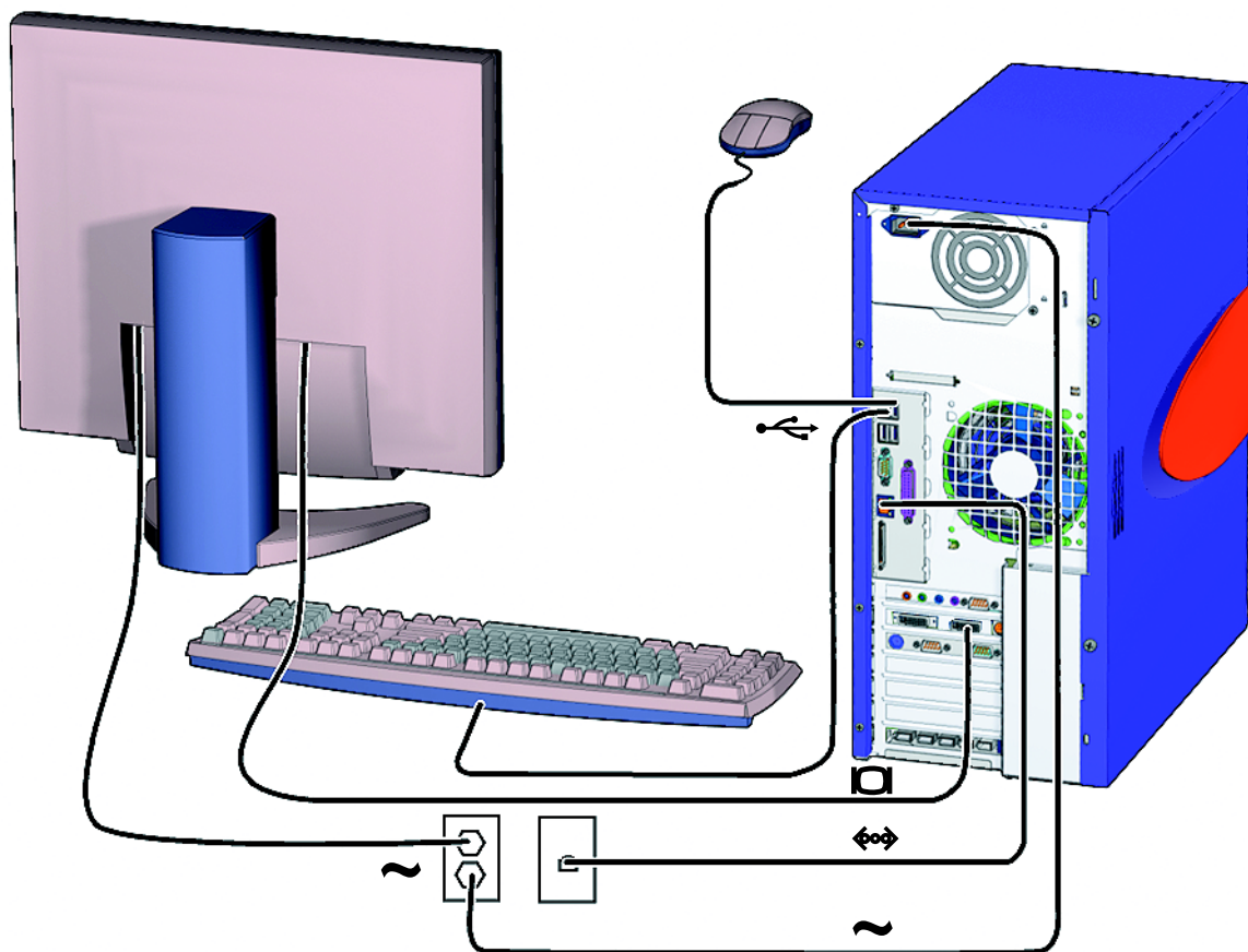
图 1-5 连接 Sun Blade 2500 工作站电缆
