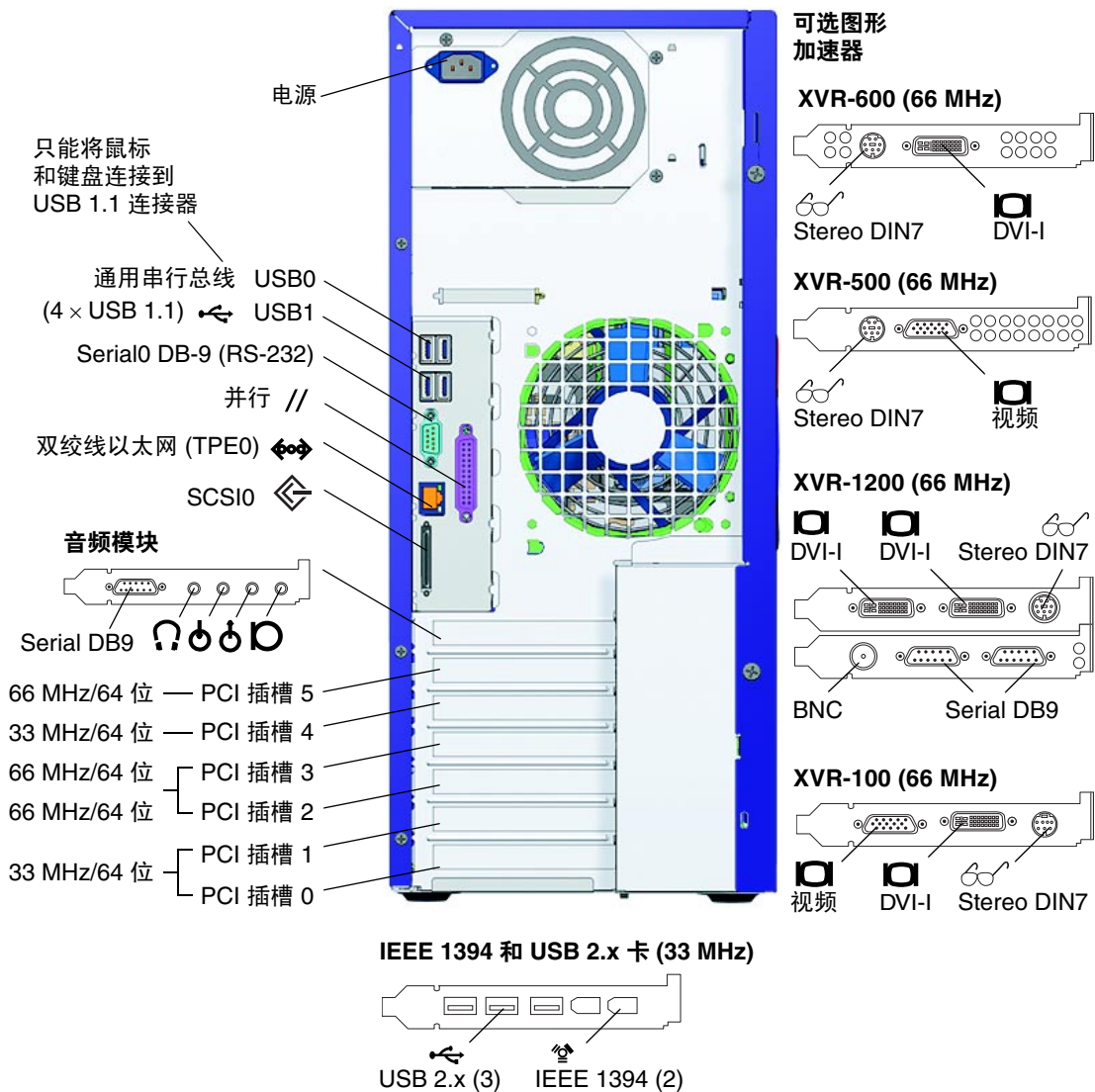
图 1-4 后面板视图
