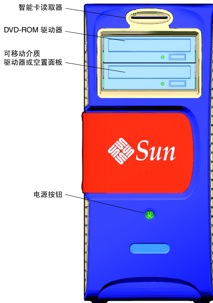
图 1-3 前面板视图
