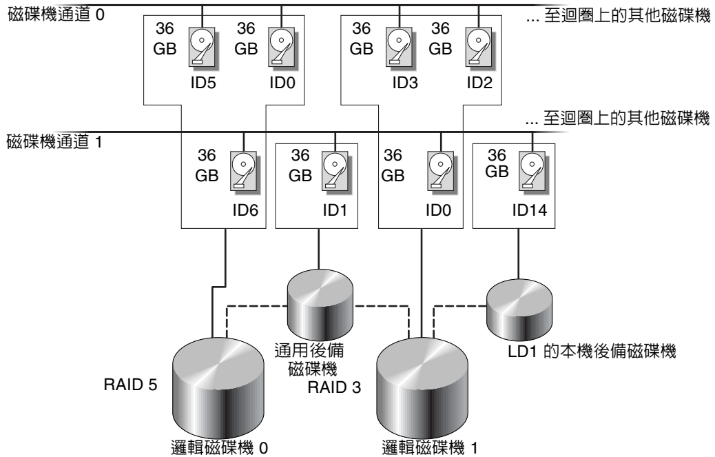
圖 5-5 邏輯配置中邏輯磁碟機與後備磁碟機的分配範例
