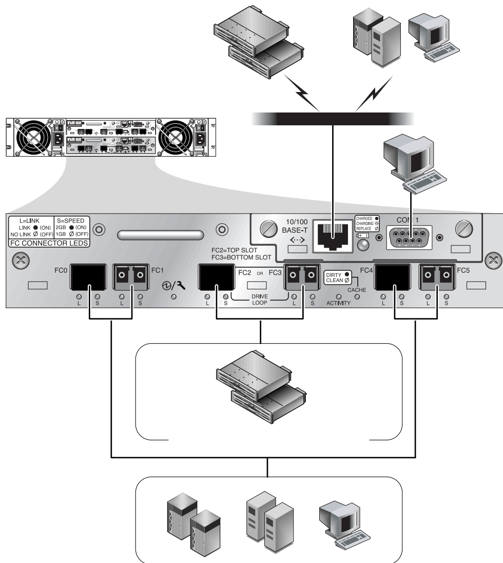
圖 4-3 雙控制器 FC 陣列背部的硬體連接
