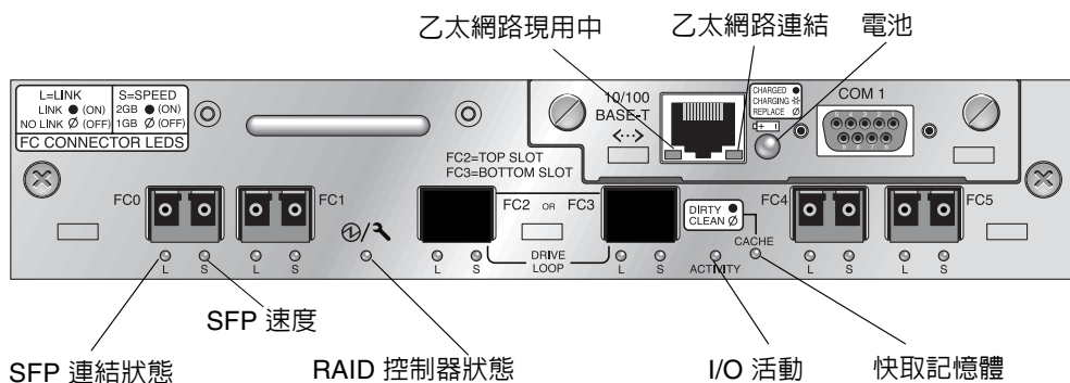
圖 6-3 I/O 控制器模組和電池模組 LED
