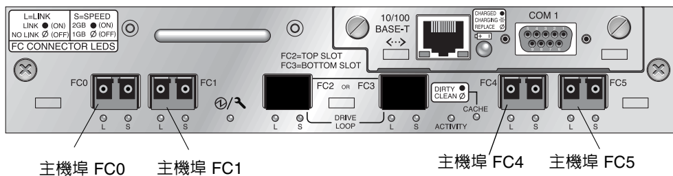
圖 4-10 預設的單控制器 SFP 位置
