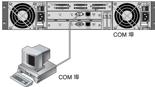
圖 G-1 RAID 陣列 COM 埠本機連接到主機系統的序列埠
