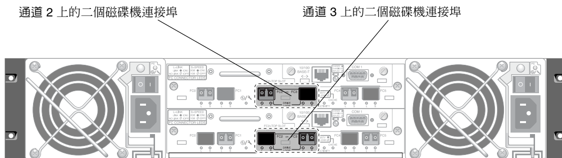
圖 4-7 雙控制器陣列中專屬的磁碟機通道 2 (在上部控制器) 和 3 (在下部控制器)
