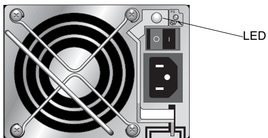
圖 6-5 交流電源和風扇模組
