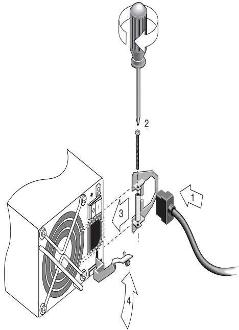
圖 4-5 安裝好的繩扣
