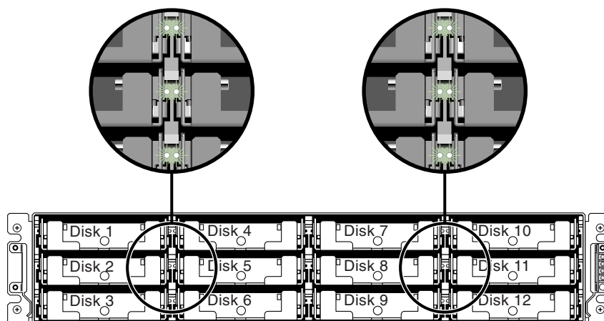
圖 8-4 閃爍所有磁碟機的 LED 以偵測有瑕疵而不會閃爍的磁碟機
