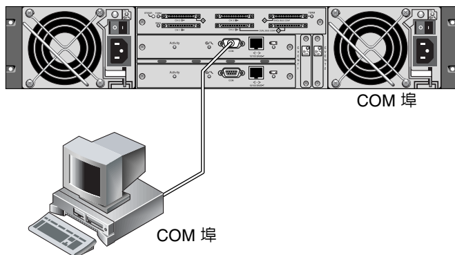
圖 E-1 RAID 陣列 COM 埠本機連接到工作站的序列埠
