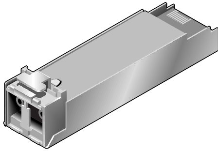
圖 4-11 用來將電纜連接至可插式 SFP 機箱埠的一般 SFP 連接器
