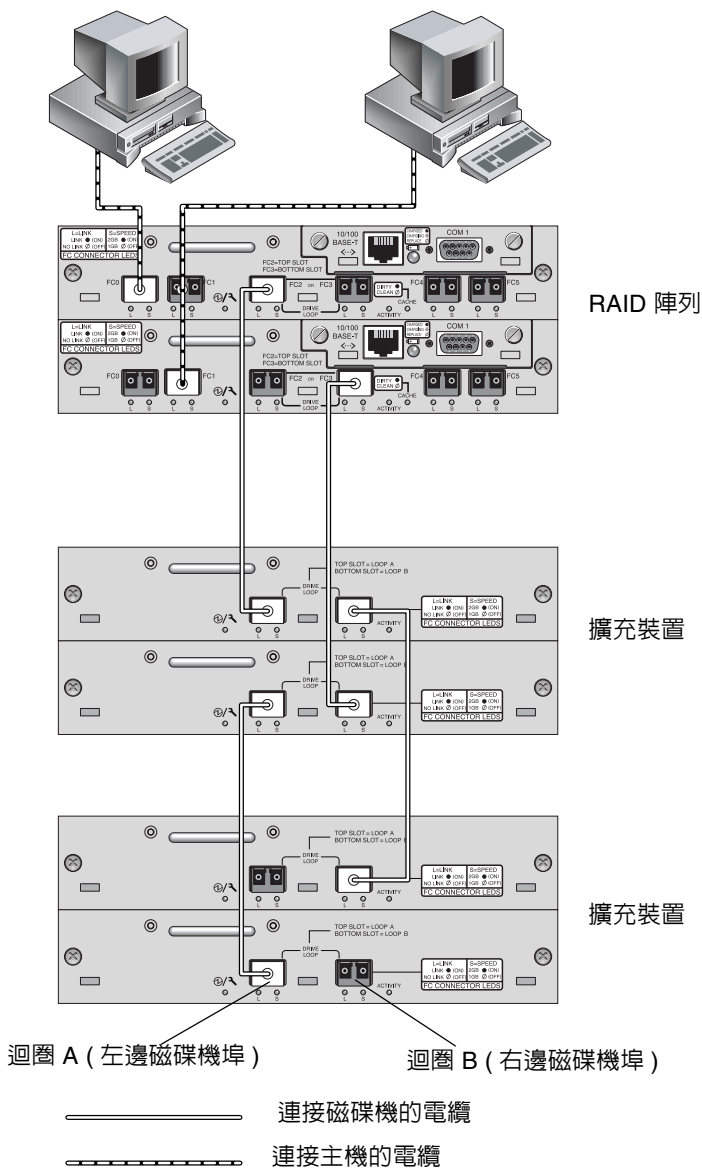
圖 4-12 連接至兩部主機和兩個擴充裝置的 RAID 陣列
