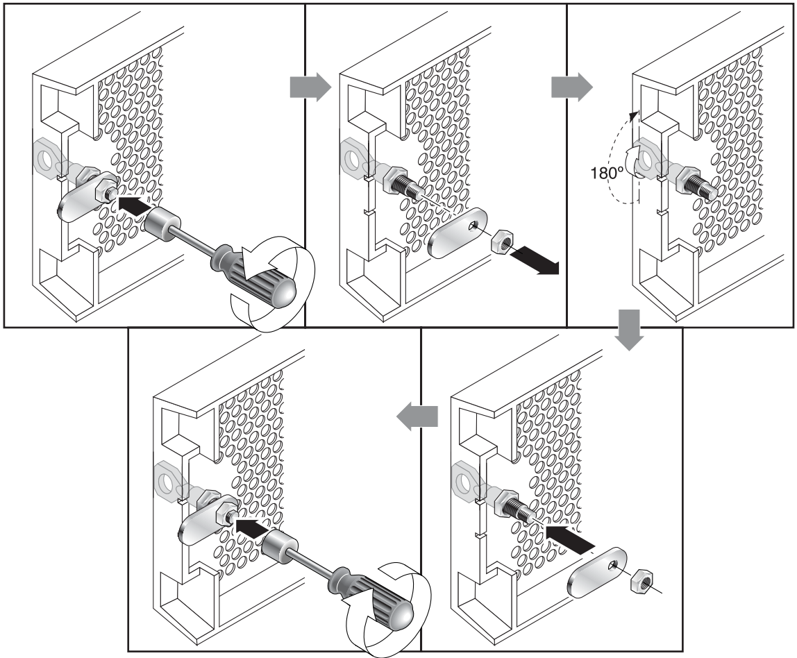
圖 4-2 變更前蓋鎖防止別人取下鑰匙的執行步驟順序
