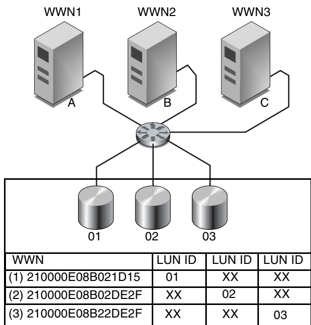
圖 5-8 LUN 篩檢範例
