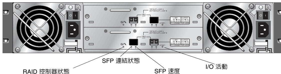
圖 6-4 擴充裝置的 I/O 擴充模組
