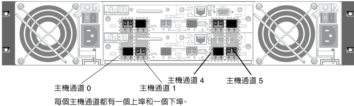
圖 4-8 雙控制器陣列中的主機通道
