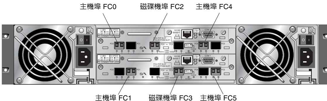
圖 4-9 預設的雙控制器 SFP 位置
