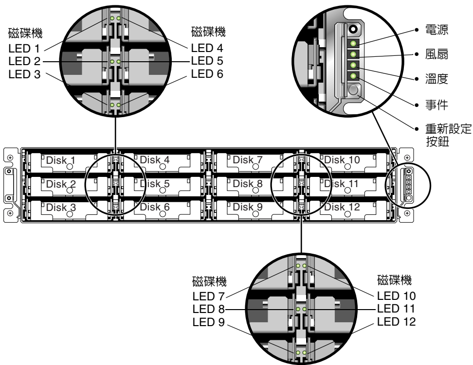
圖 6-1 前面板 LED
