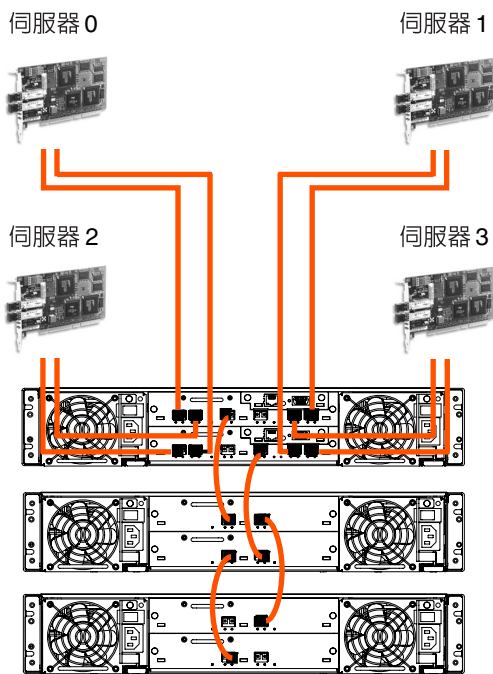
圖 5-2 包含四台伺服器、一個雙控制器陣列和兩個擴充裝置的 DAS 配置
