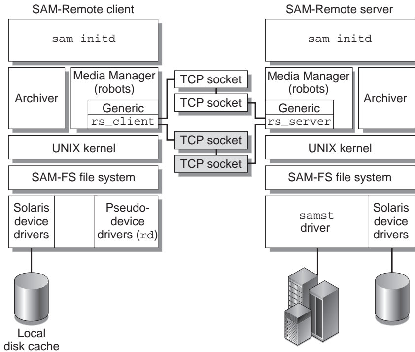
FIGURE 1-2 Interactions entre serveur et client Sun SAM-Remote
