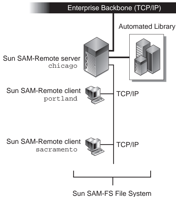
FIGURE 2-1 Exemple de configuration de Sun SAM-Remote
