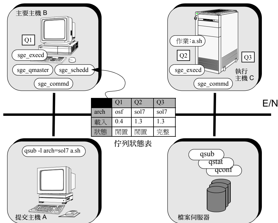
圖 1-3 Sun Grid Engine，企業版系統的組件互動
