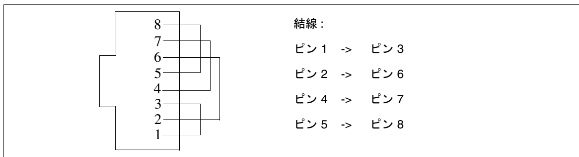
図 A-16 Gigabit Ethernet 用 TPE ループバックケーブルの結線
