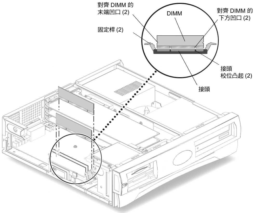
圖 4-7 安裝 DIMM
