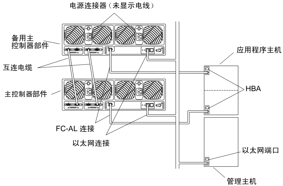
图 2-10 电缆已完全接好的伙伴组（企业配置）
