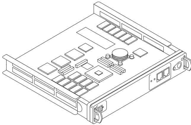
图 B-3 Sun StorEdge T3+ 阵列控制卡
