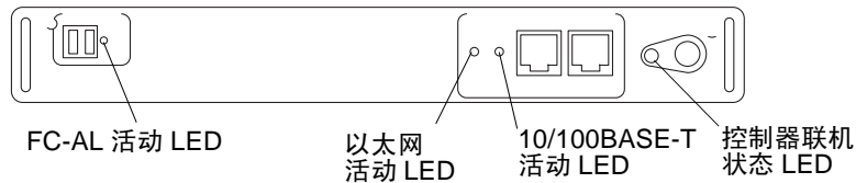
图 4-5 Sun StorEdge T3+ 阵列控制器卡 LED
