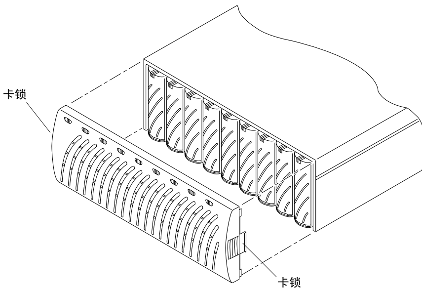
图 5-1 拆卸前面板
