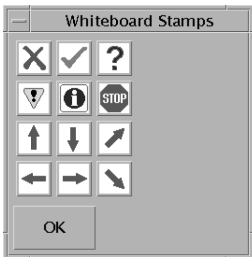
FIGUR 2-9 Fönstret Whiteboard-stämplar
