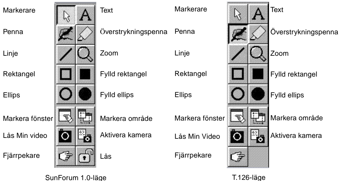
FIGUR 2-5 Whiteboards verktygsfält
