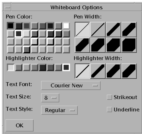
FIGUR 2-7 Fönstret Whiteboard-inställningar
