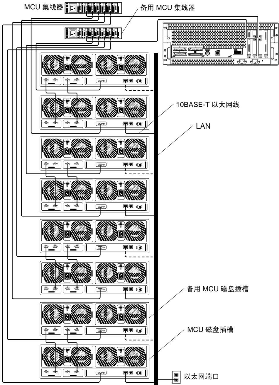
图 1 Sun StorEdge N8400 Filer 的最大配置
