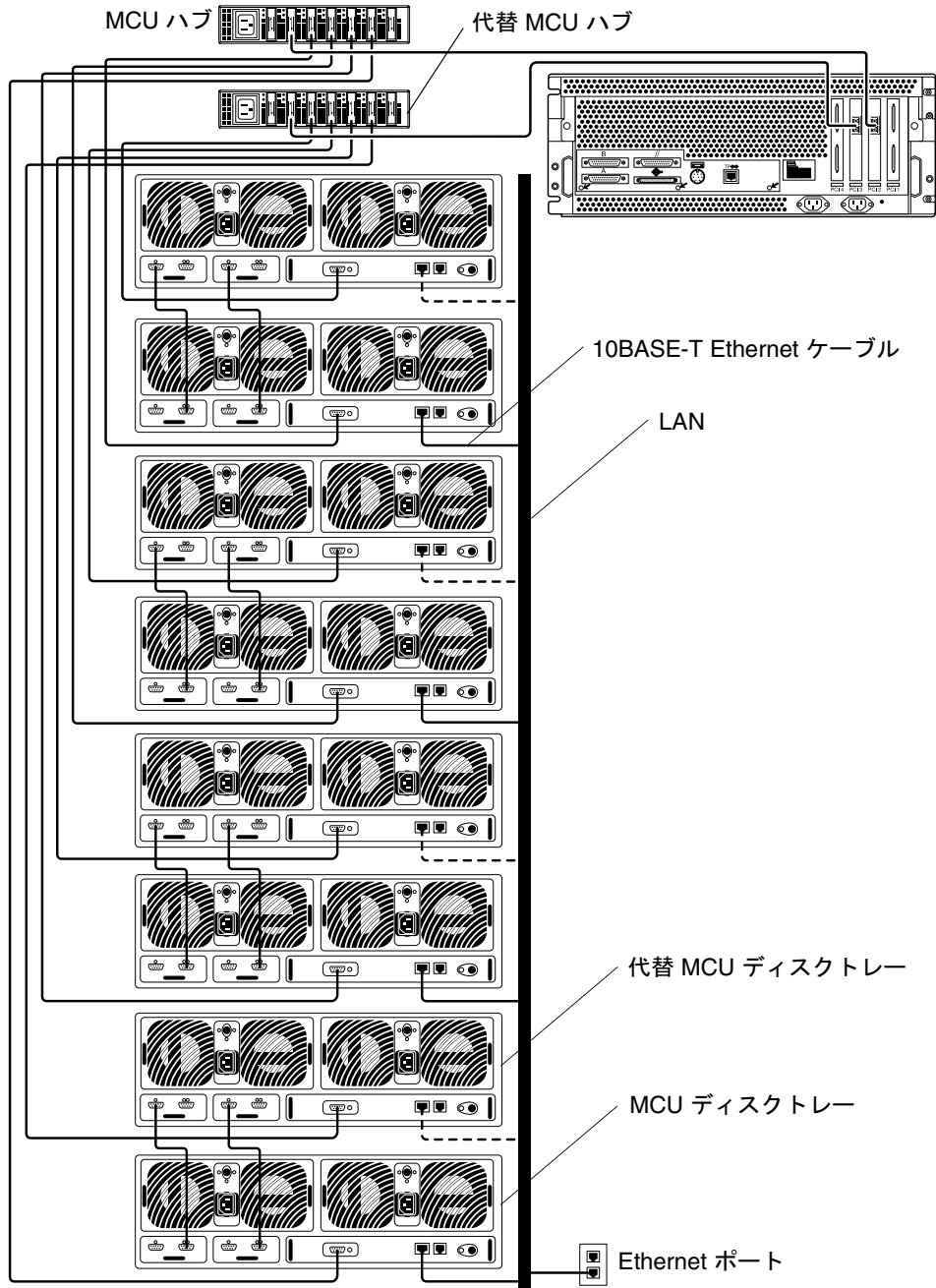
図 1 Sun StorEdge N8400 Filer の最大構成
