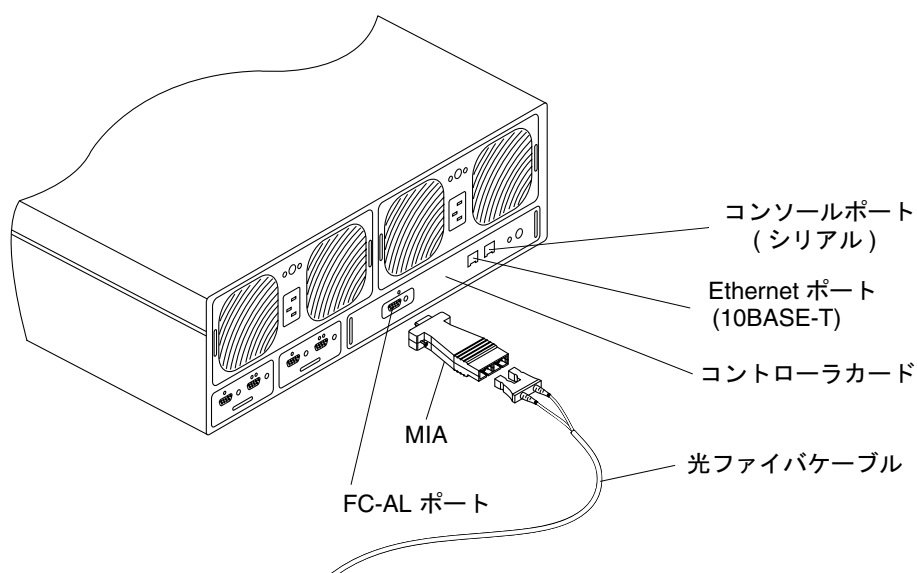
図 2 ディスクトレイの背面パネルの詳細
