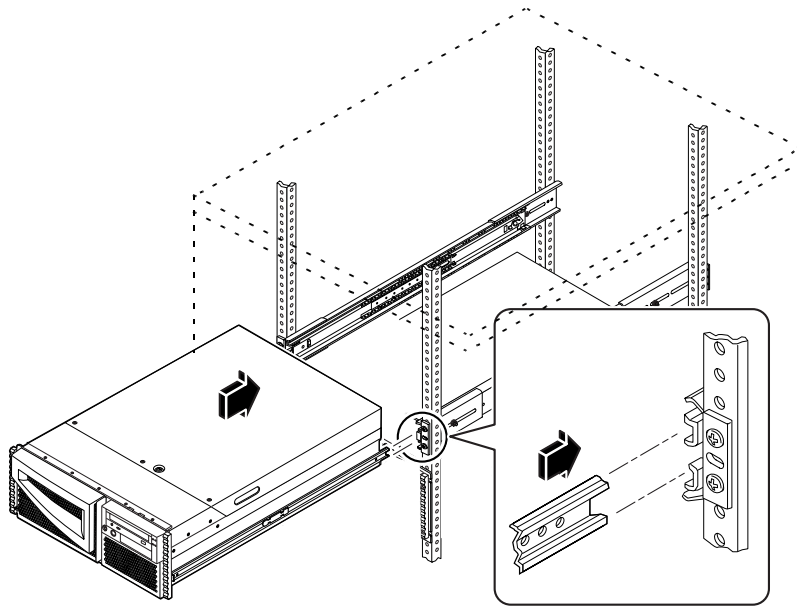
그림 4 Sun Enterprise 420R Server 설치
