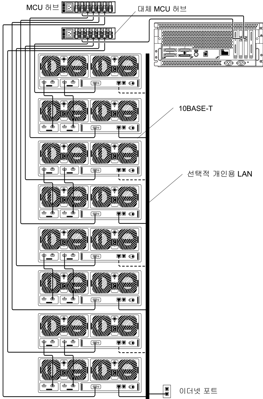
그림 9 Sun StorEdge N8400 Filer를 위한 최대 구성
