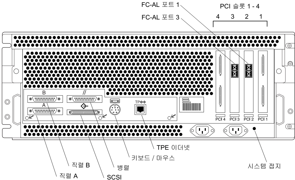
그림 8 Sun Enterprise 420R Server 뒤쪽 패널 상세도 및 연결
