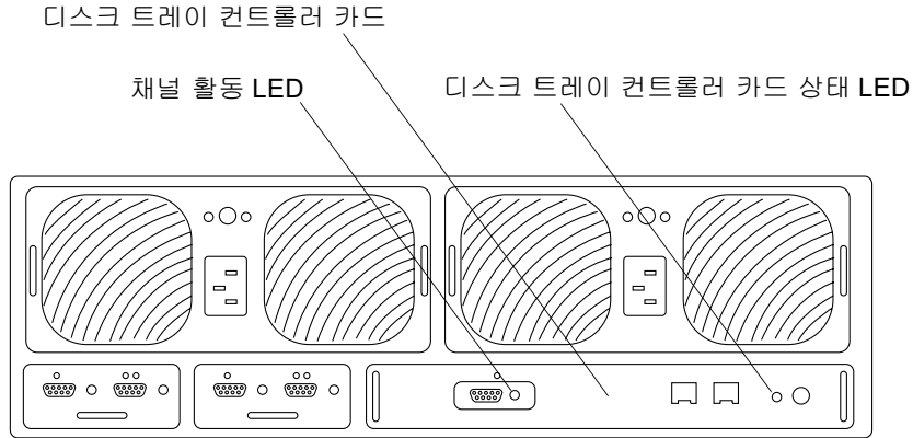
그림 12 Sun StorEdge T3 디스크 트레이의 뒤쪽
