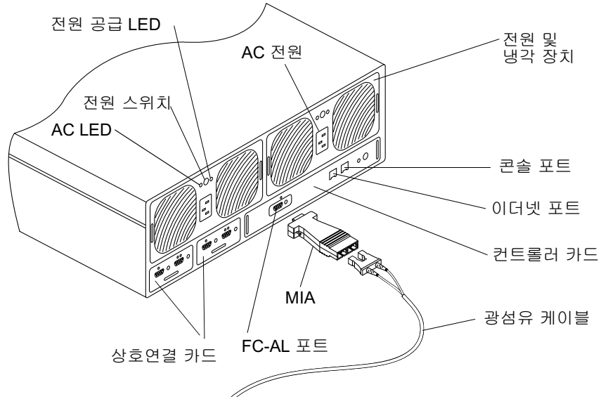
그림 6 디스크 트레이 뒤쪽 패널 상세도
