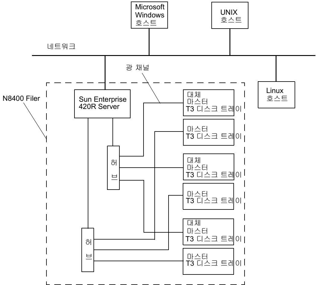
그림 2 Sun StorEdge N8400 Filer 시스템 예
