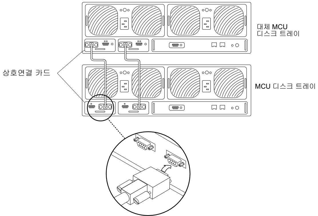
그림 5 상호연결 케이블 연결
