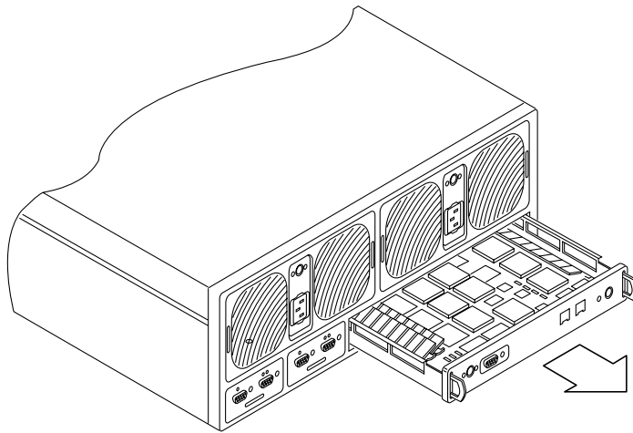
그림 13 SunStorEdge T3 컨트롤러 카드 제거
