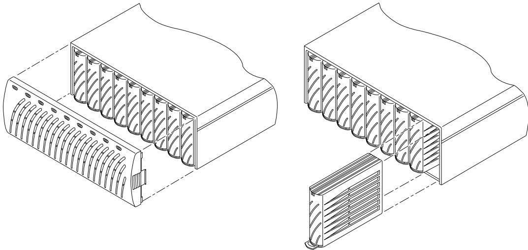
그림 11 디스크 트레이 앞쪽 패널 및 디스크 드라이브 제거
