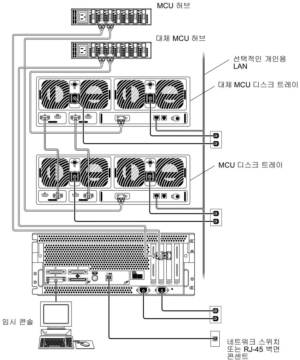
그림 7 설정 목적을 위한 Sun Enterprise 420R Server와 디스크 트레이의 파트너 그룹 사이의 연결
