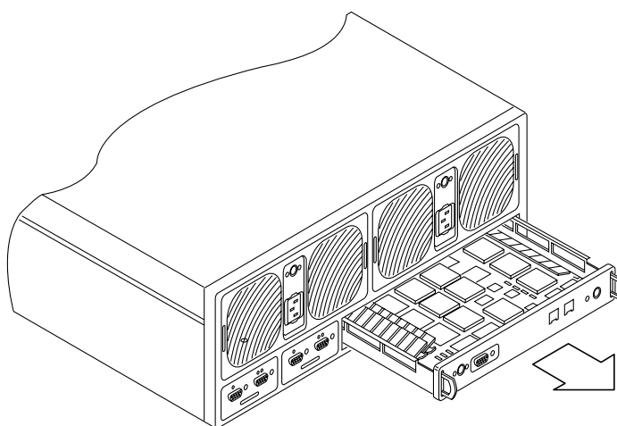
図 13 SunStorEdge T3 コントローラカードの取り外し
