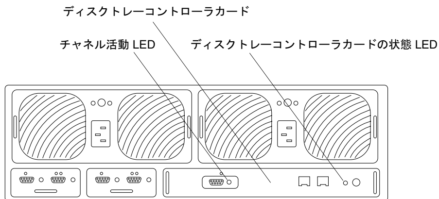
図 12 Sun StorEdge T3 ディスクトレイの背面
